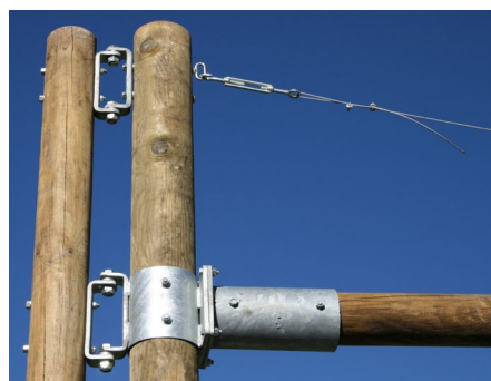
Détail Ferrures et câble de tension
