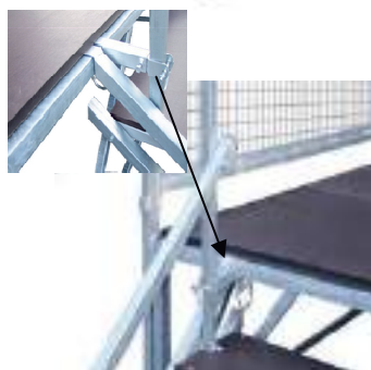
Système de fixation de l'escalier au podium
